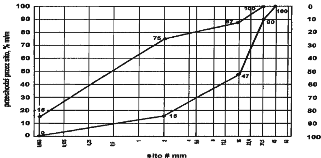
Rys.1 - Mieszanka niezwiązana 0/31,5 mm
