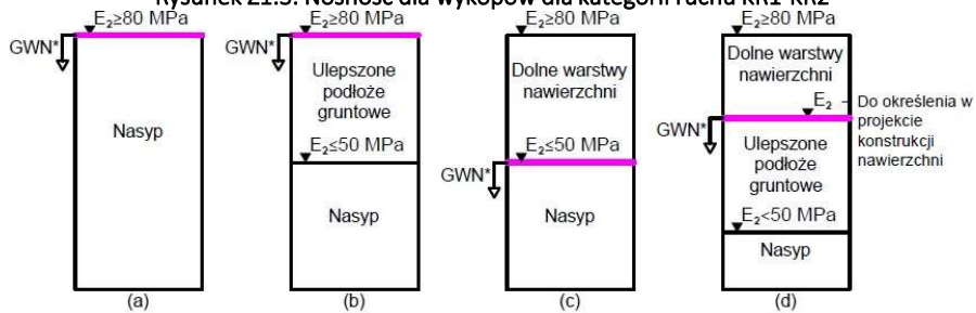
Rysunek Z1.3. Nośność dla wykopów dla kategorii ruchu KR1-KR2
