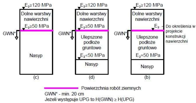
Rysunek Z1.5. Nośność dla nasyków dla kategorii ruchu KR5-KR7
