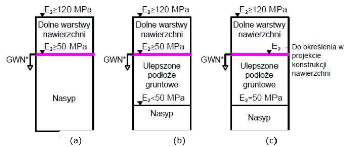
Rysunek Z1.6. Nośność dla wykopów dla kategorii ruchu KR5-KR7
