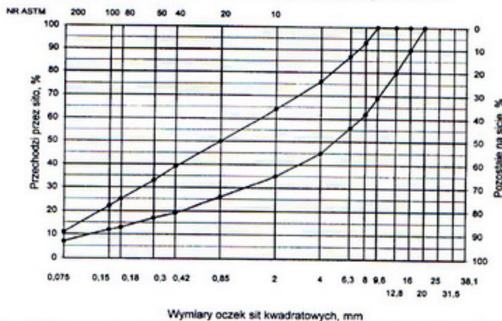
Rys. 2. Krzywe graniczne uziarnienia mieszanki mineralnej BA od 0 do 16mm, od 0 do 12,8 mm do warstwy ścieralnej nawierzchni drogi o obciążeniu ruchem KRI lub KR2
