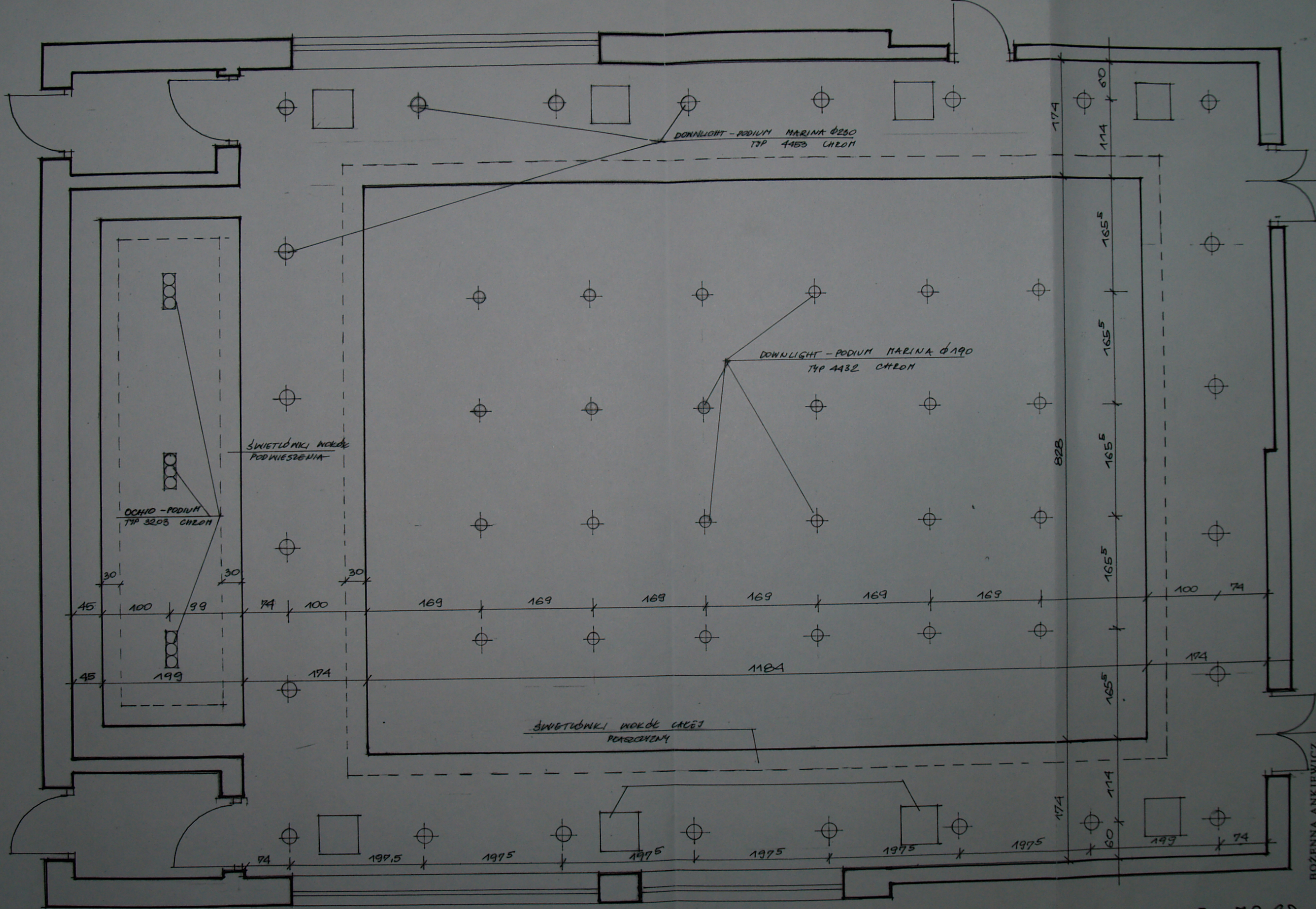
RZUT SUFITU PODWIESZANEGO 1:30
