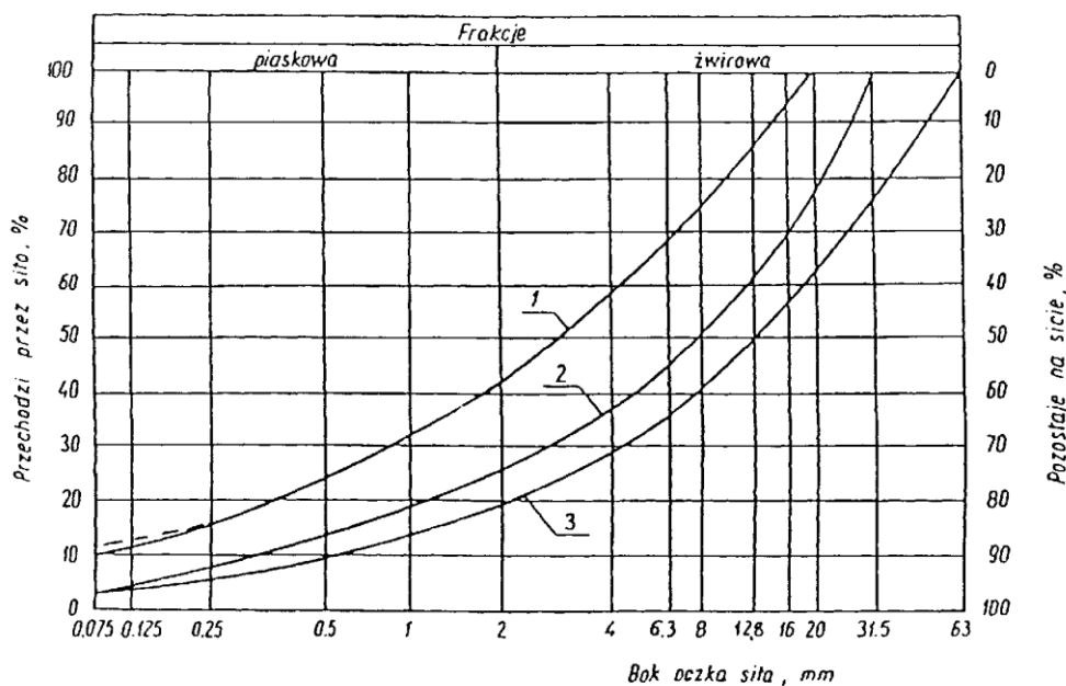
Rysunek 1. Pole dobrego uziarnienia kruszywa przeznaczonych na podbudowy wykonywane metoda stabilizacji mechanicznej
