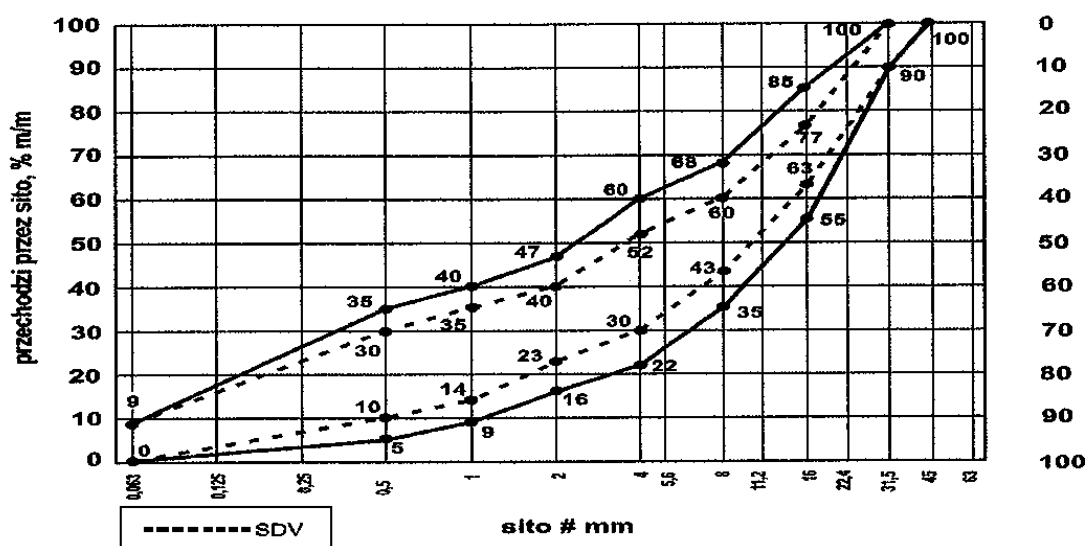
Rys. 1. Krzywe graniczne uziarnienia mieszanki kruszywa niezwiązanego 0/31,5 mm warstw podbudowy zasadniczej do
